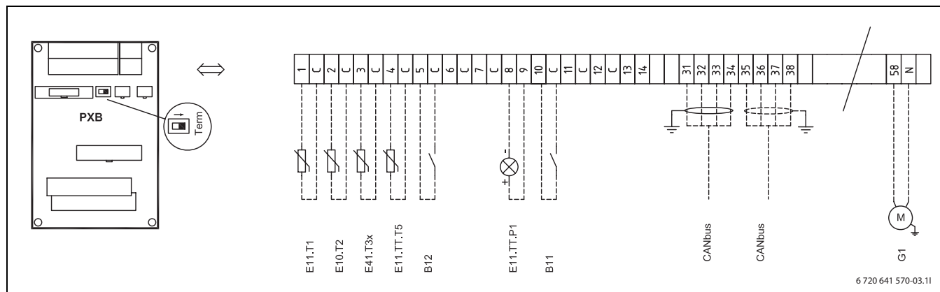
Bild 49 Externa anslutningar
