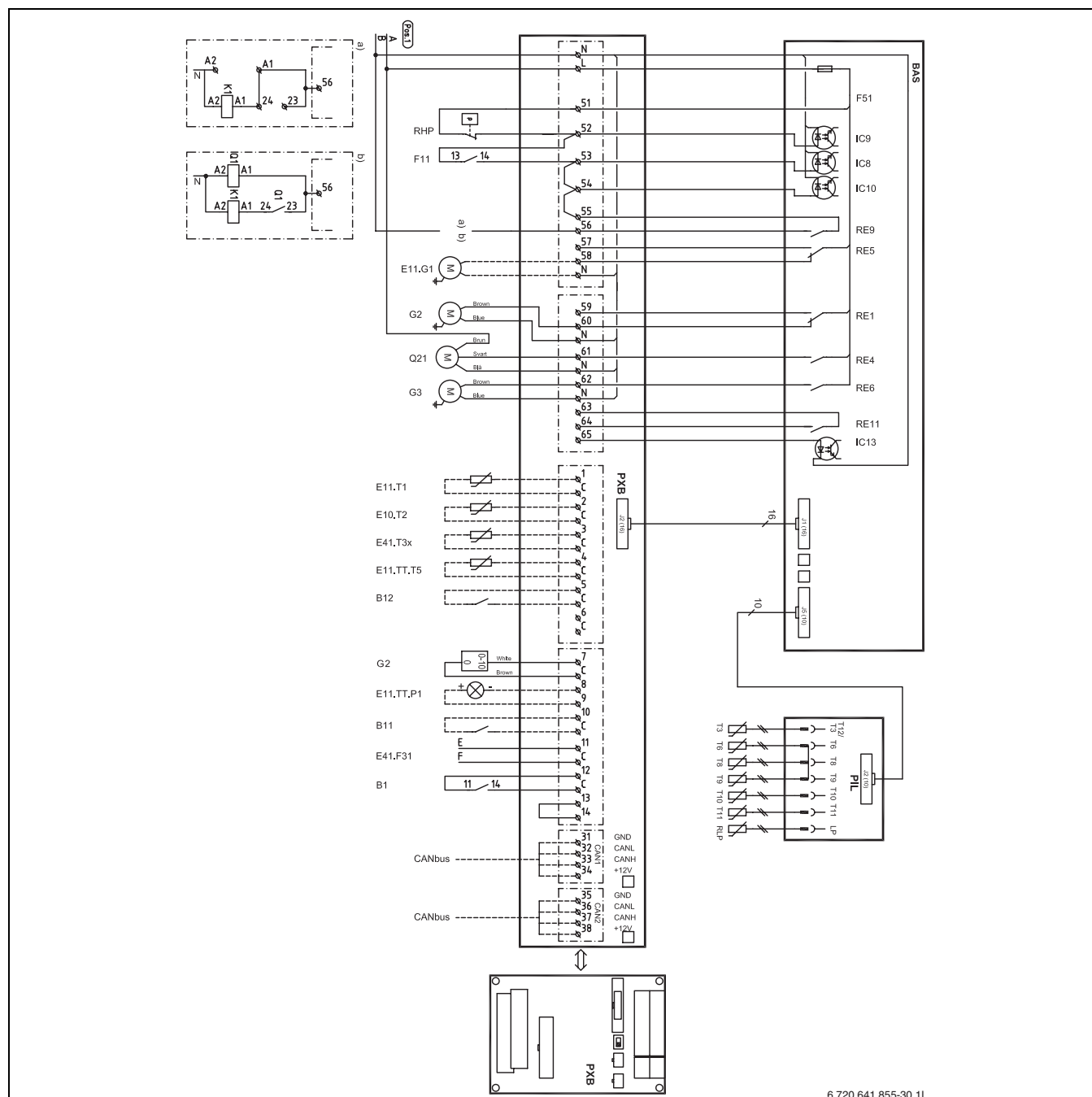
Bild 48 Komplettschema anslutningar
