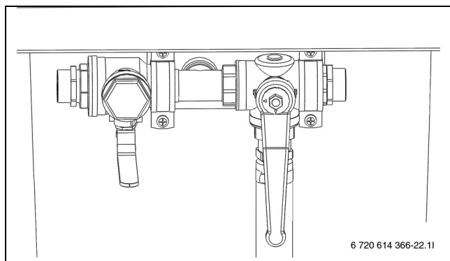
Bild 38 Påfyllnadsstation i blandningsläge
