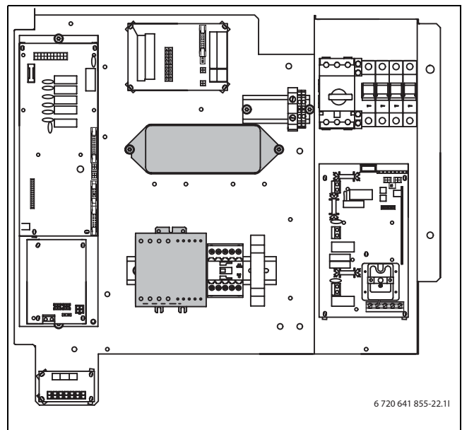
Bild 31 Montera mjukstarten samt filter.
