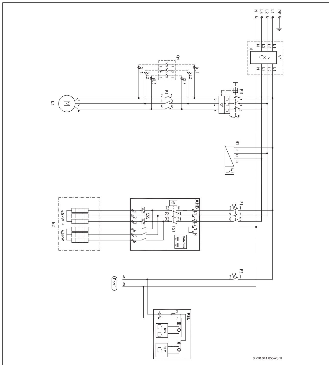
Bild 46 Internt elschema
