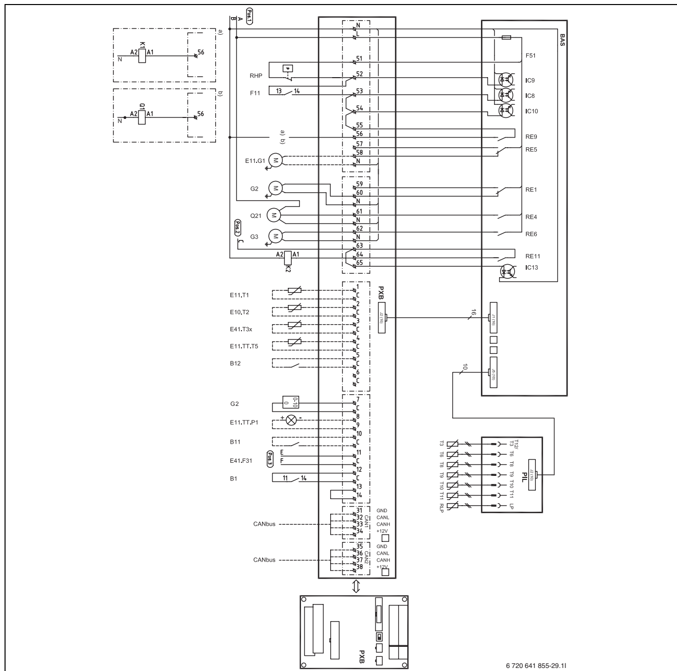
Bild 47 Komplette elschema anslutningar
