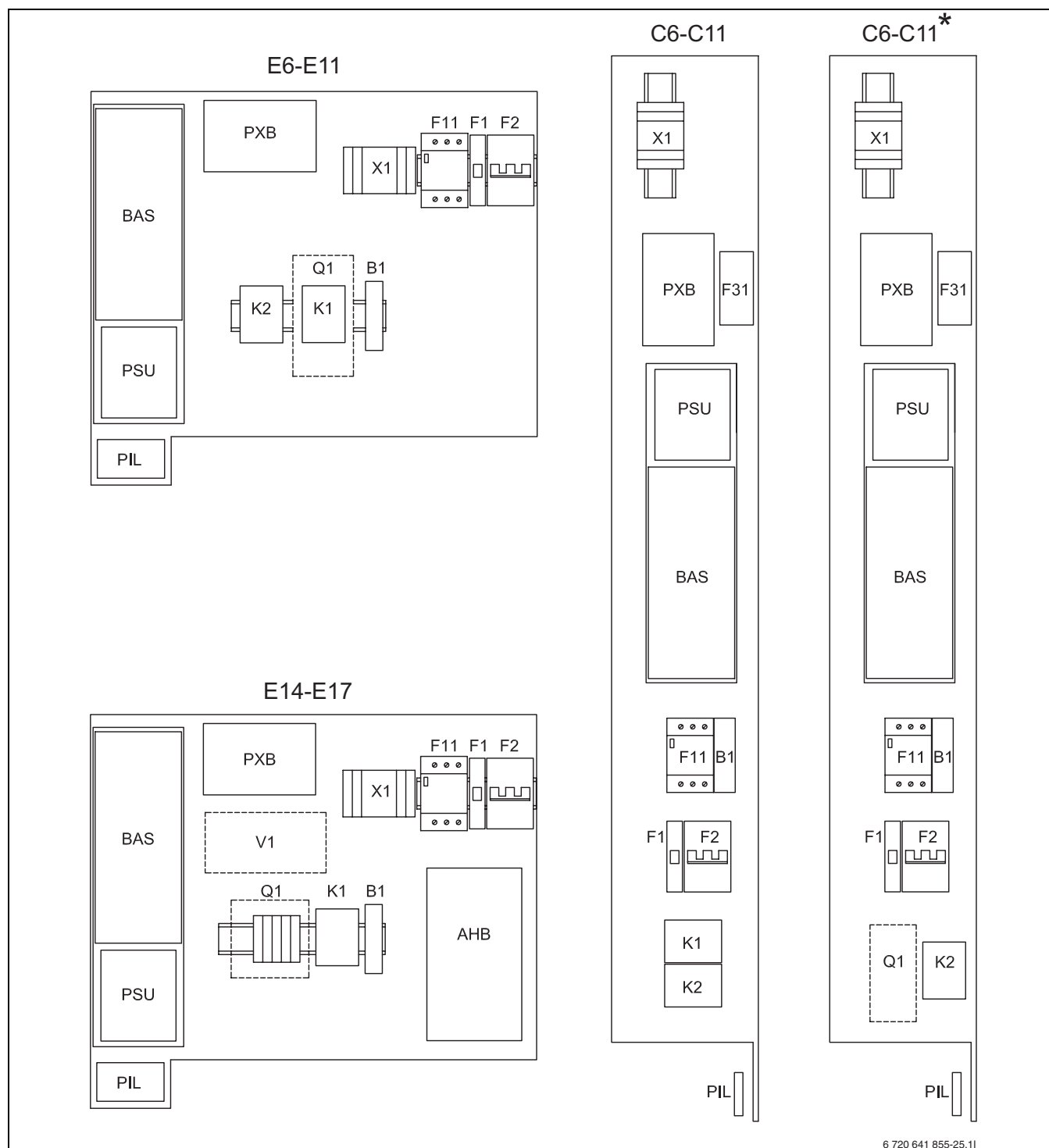
Bild 42 Översikt kretskort
