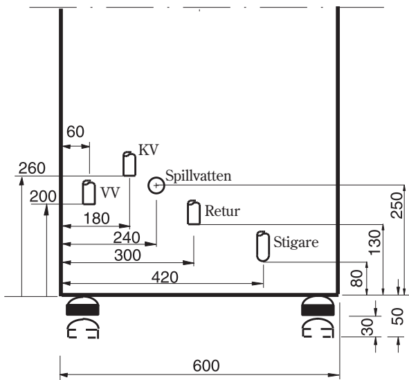
Vy framifrån
