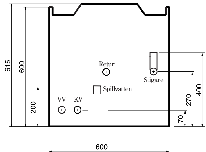
Vy uppifrån
