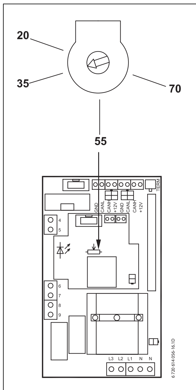
Bild 47 AHB-kort
