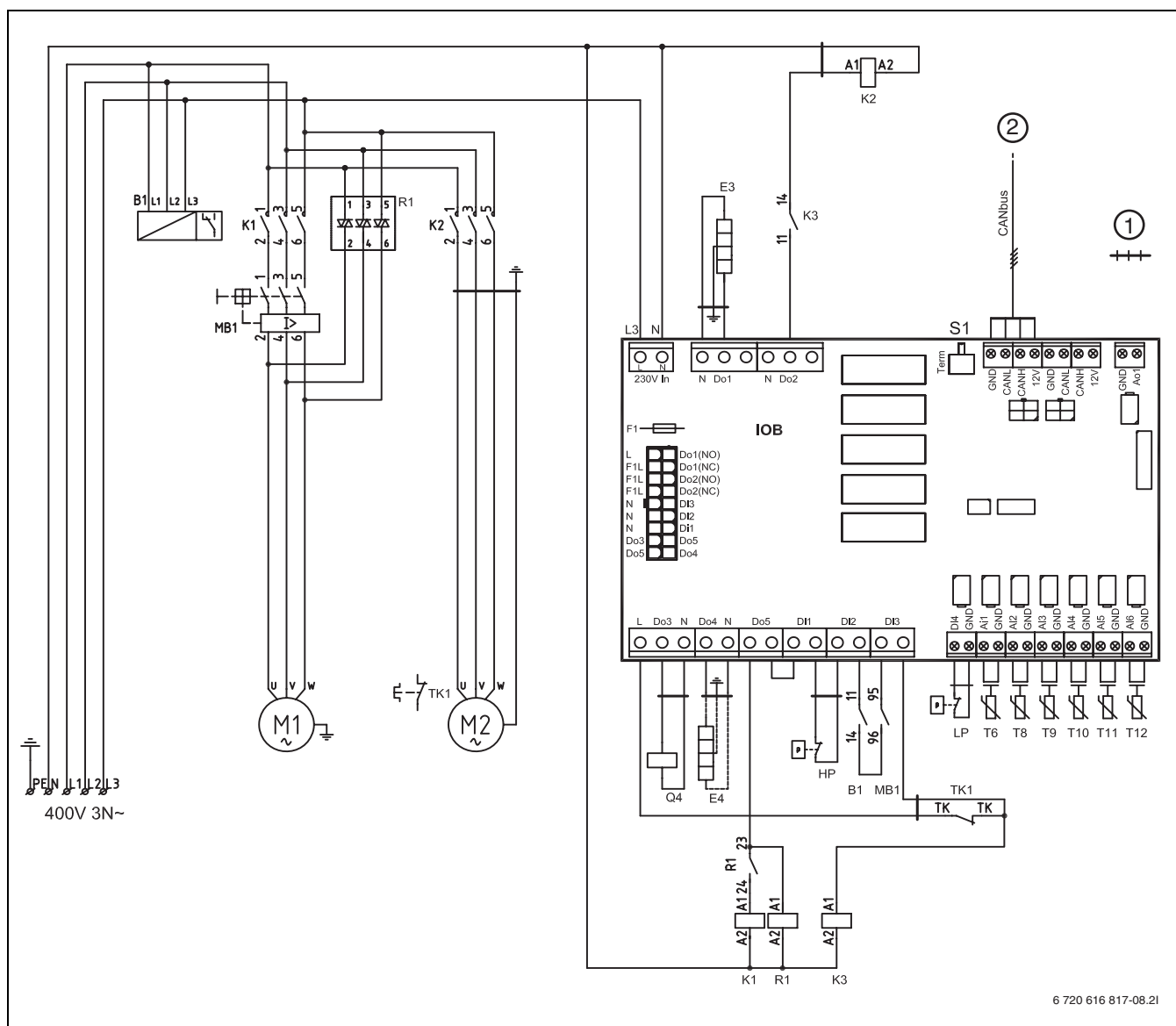
Bild 49 Elschema Air 120-150
