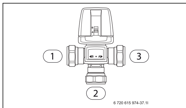
Bild 38 Växelventil
