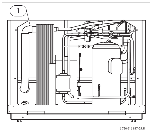
Bild 45 Värmepump
