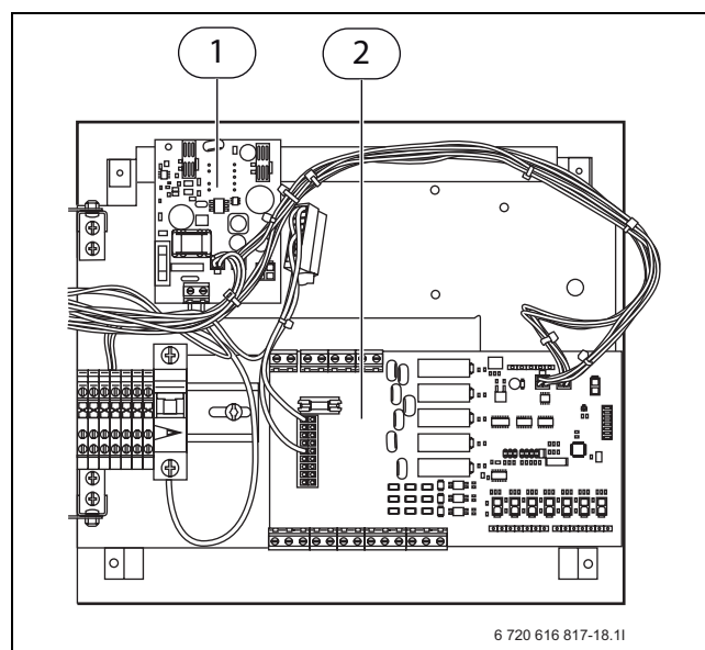
Bild 21 Styrskåp
