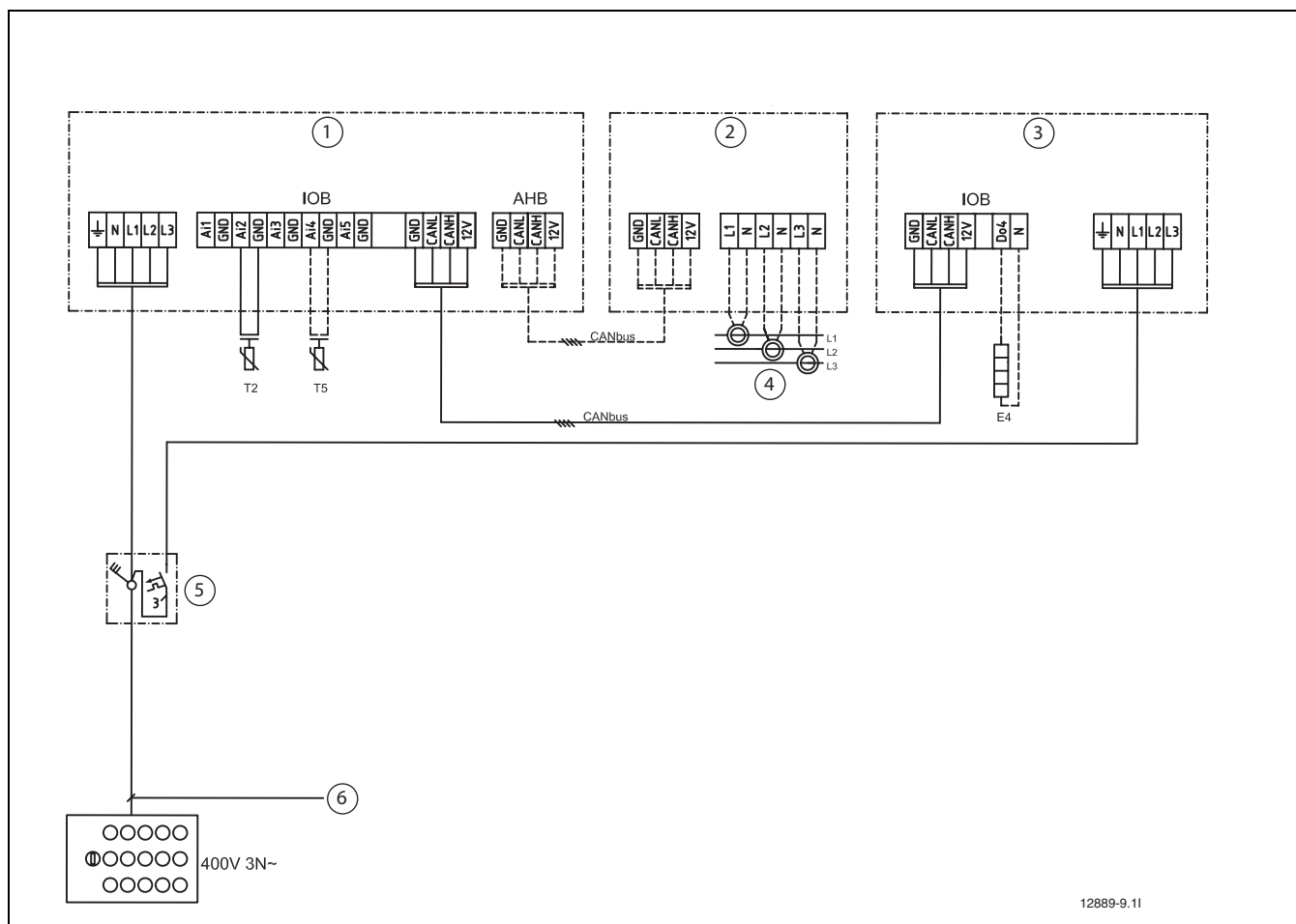
Bild 55 Anslutningsschema värmepump - kombimodul
