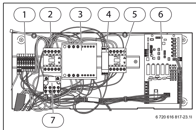
Bild 16 Ellåda Air 120-150
