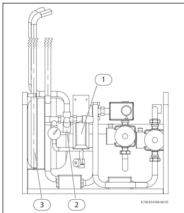
Bild 28 Elpanna framsida
