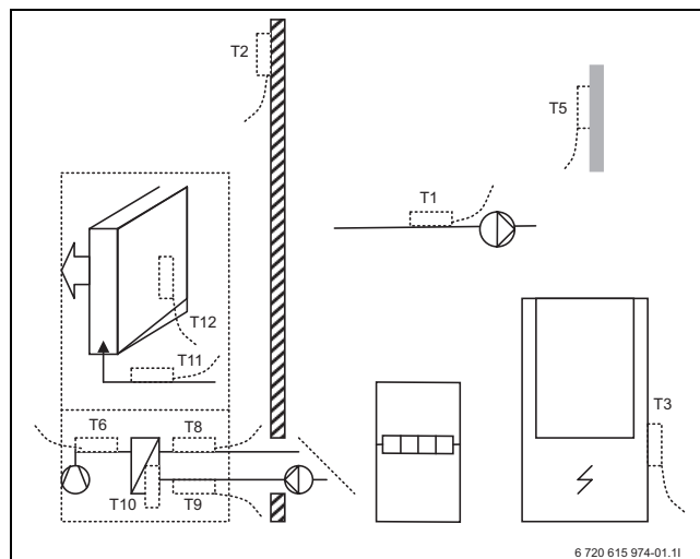
Bild 8 Air 50-150 - Elkassett.
