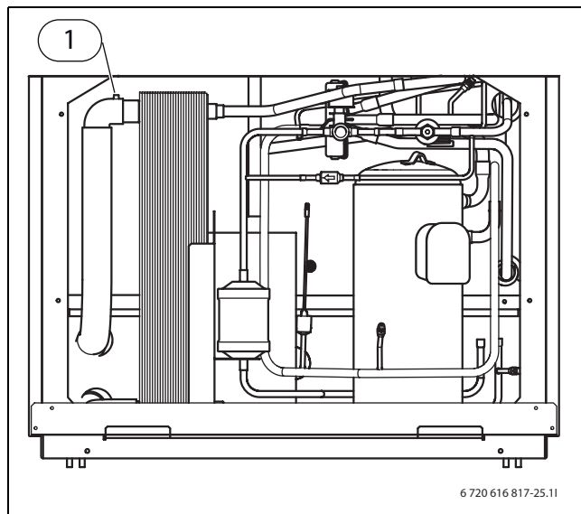
Bild 87 Värmepump
