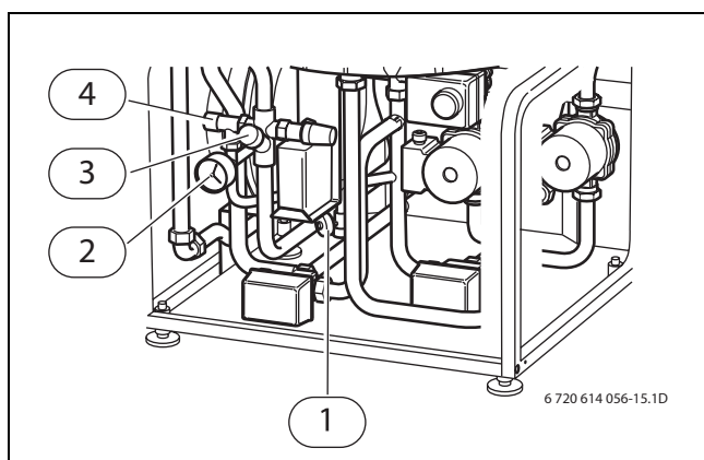
Bild 43 Kopplingsutrymme elpanna
