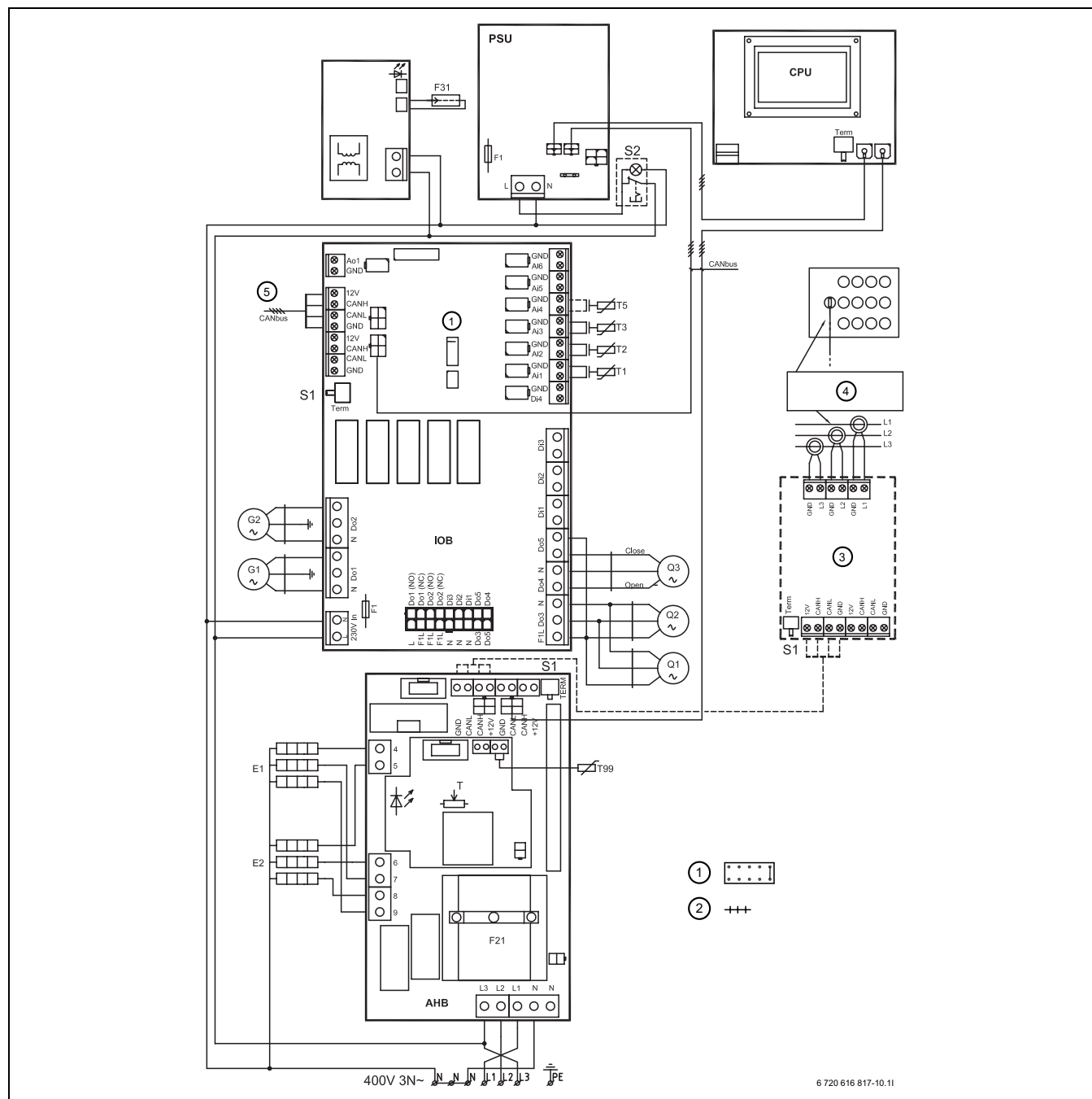
Bild 51 Elschema 290 A/W
