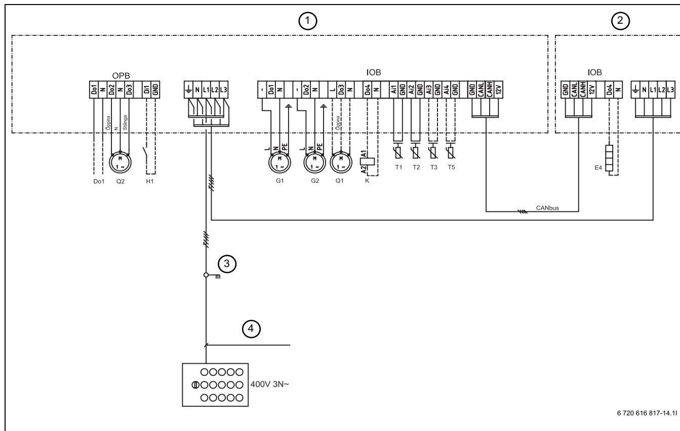
Bild 62 Anslutningsschema värmepump - shuntat tillskott.
