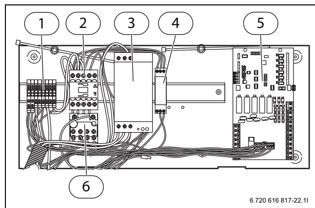
Bild 15 Ellåda Air 50-90
