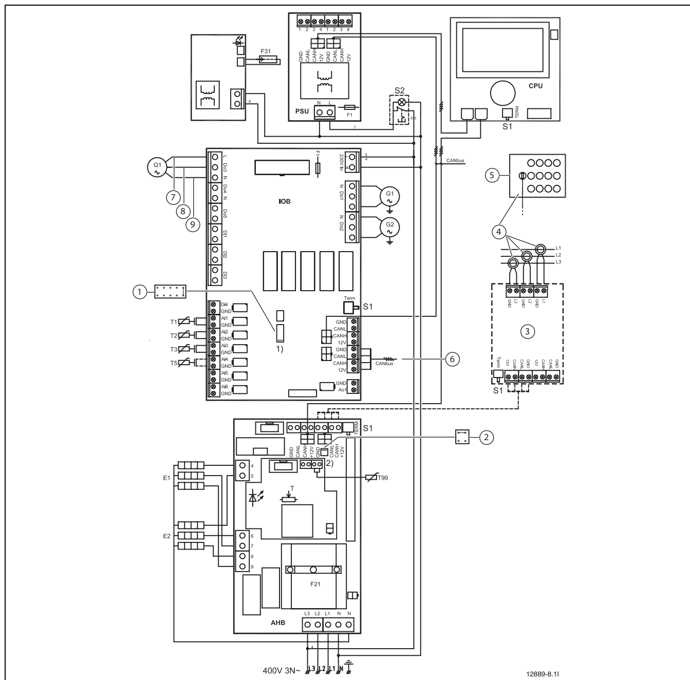
Bild 54 Elschema kombimodul
