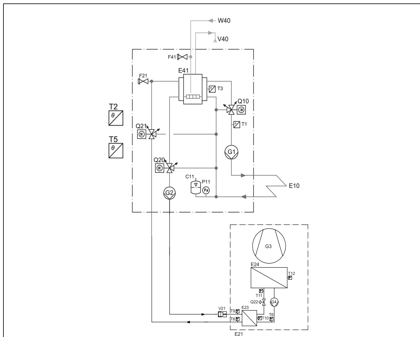
Bild 39 Värmepump med elpanna
