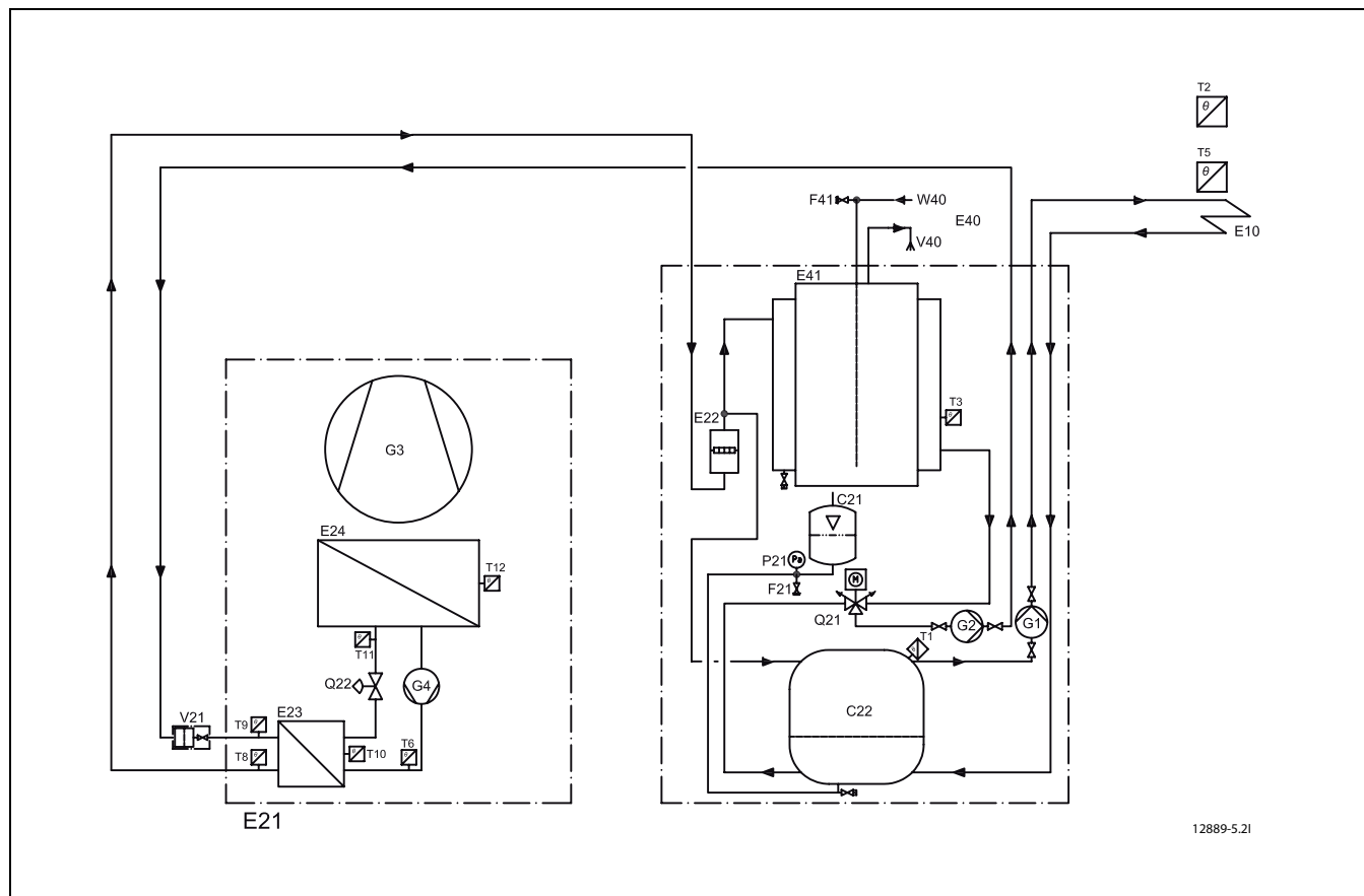
Bild 40 Värmepump med kombimodul 200-300 A/W
