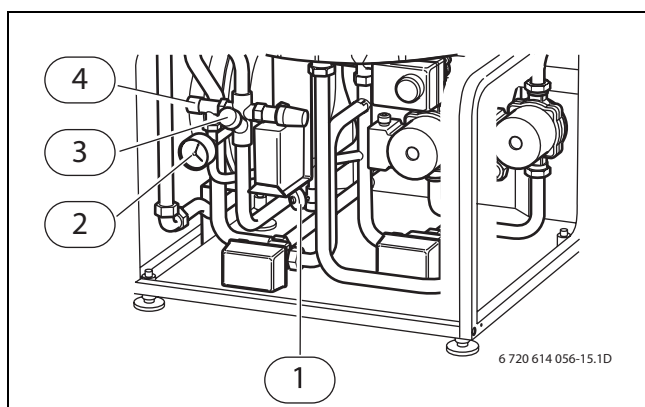
Bild 86 Elpanna
