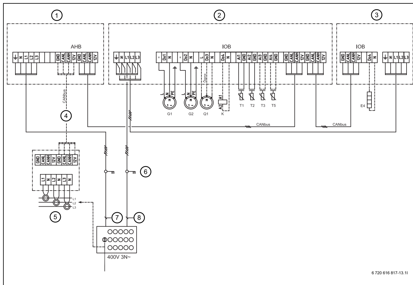
Bild 59 Anslutningsschema värmepump - elkassett.
