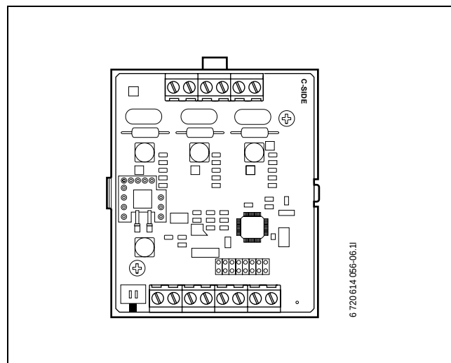
Bild 24 Effektvaktskort (tillval)
