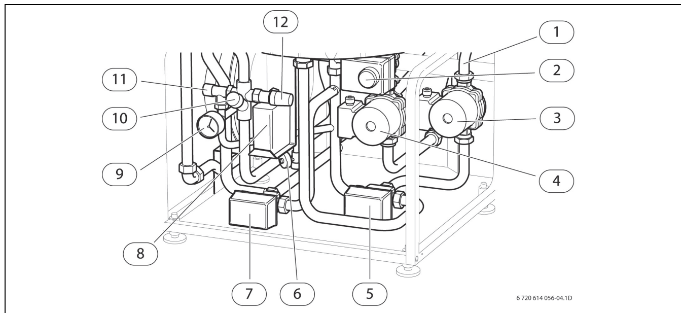
Bild 17 Kopplingsutrymme elpanna
