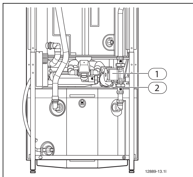
Bild 99 Kopplingsutrymme Kombimodul
