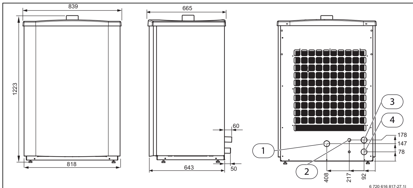
Bild 25 Mått Air 50-90
