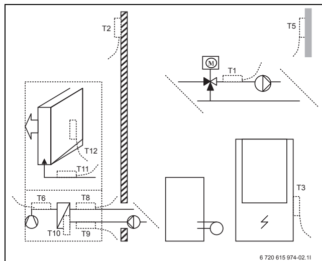
Bild 9 Air 50-150 - Shuntat tillskott.
