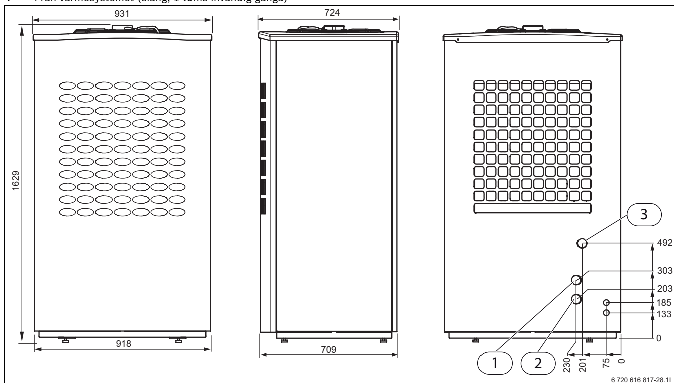
Bild 26 Mått Air 120-150
