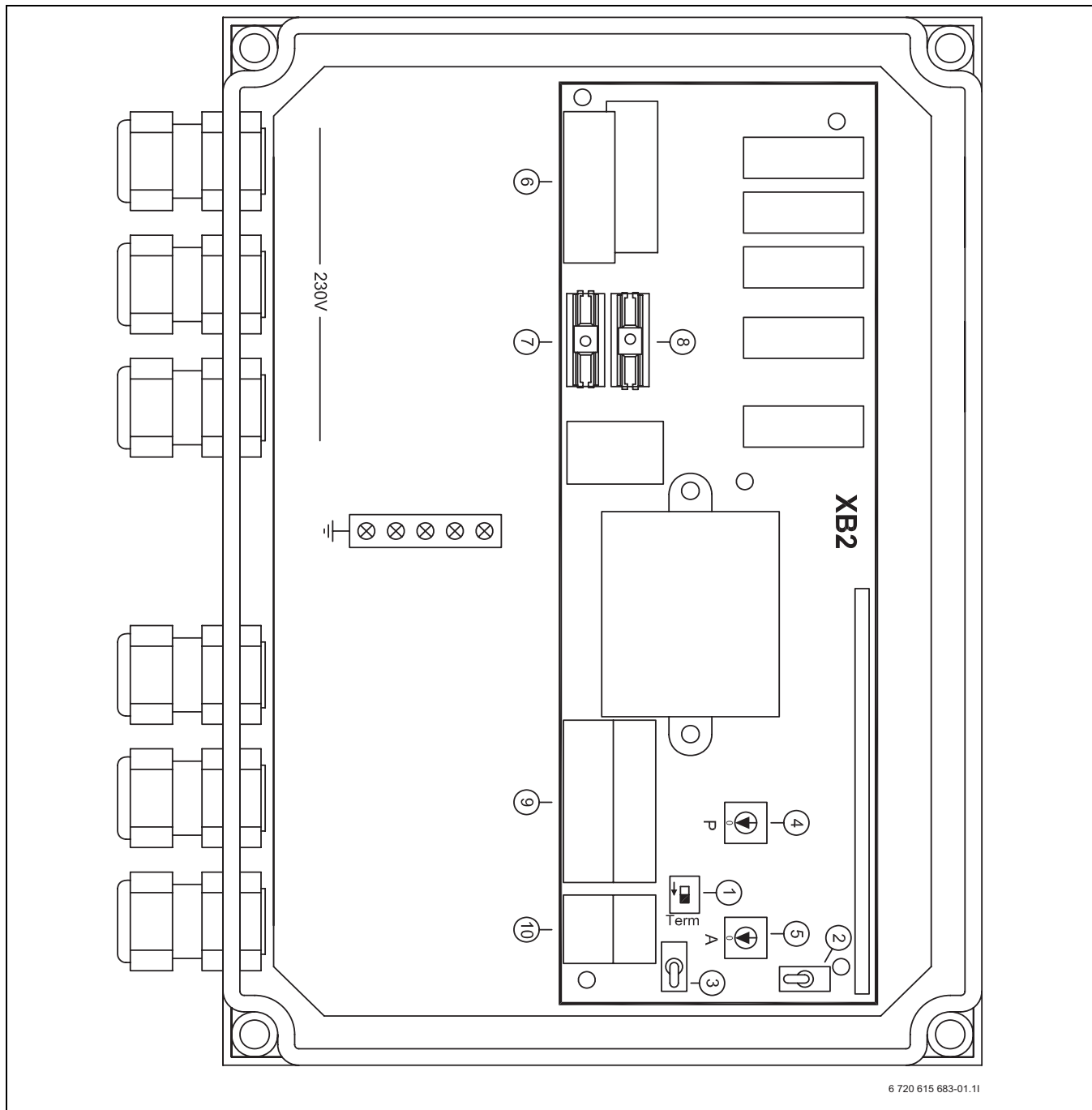
Bild 8 Shuntmodul XB2
