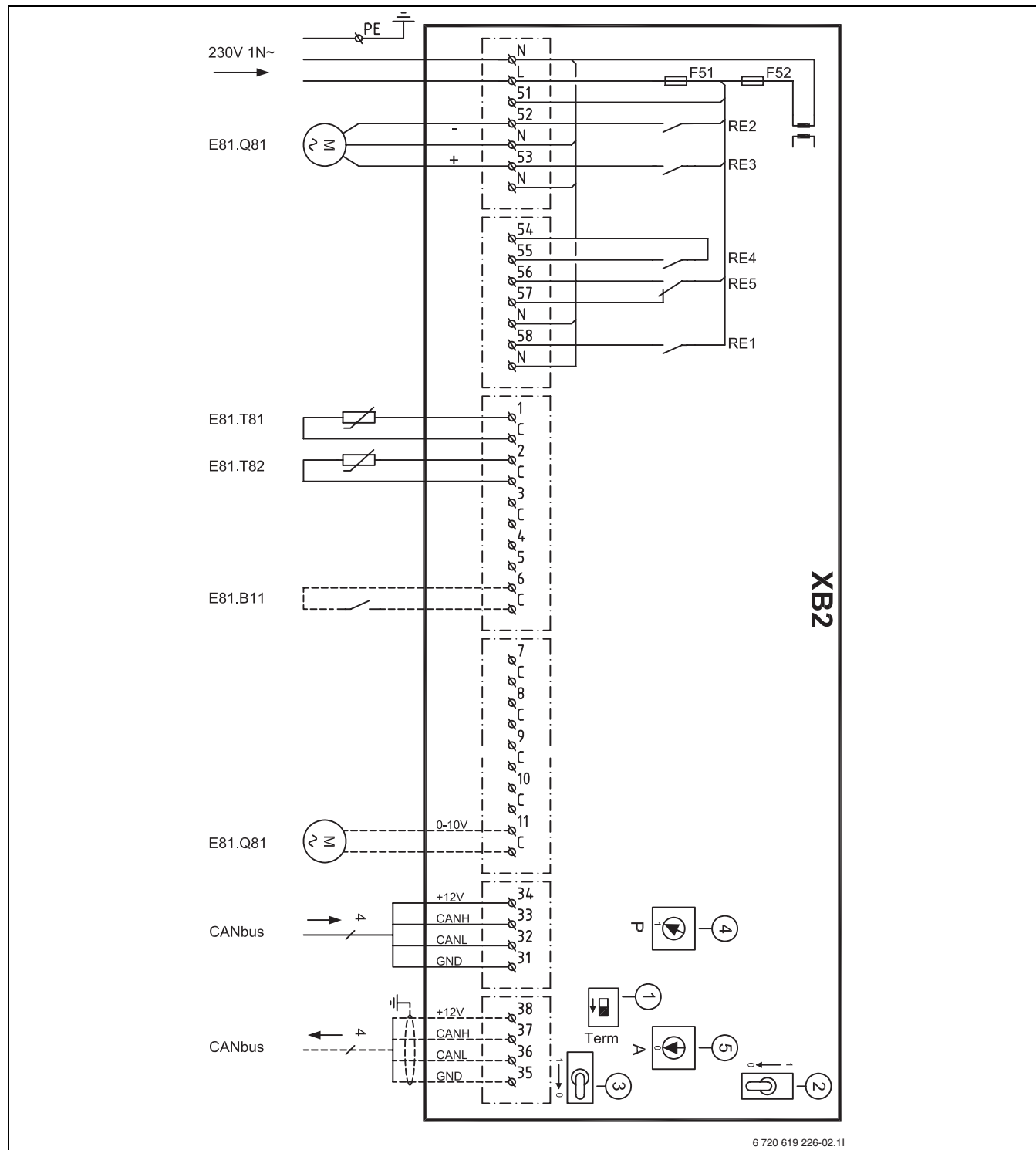
Bild 12 Elschema poolstyrning
